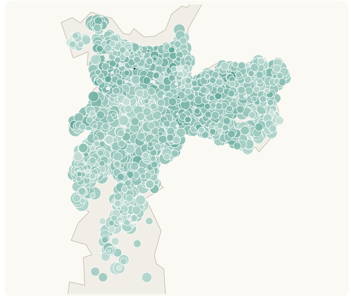
% dos válidos no local
