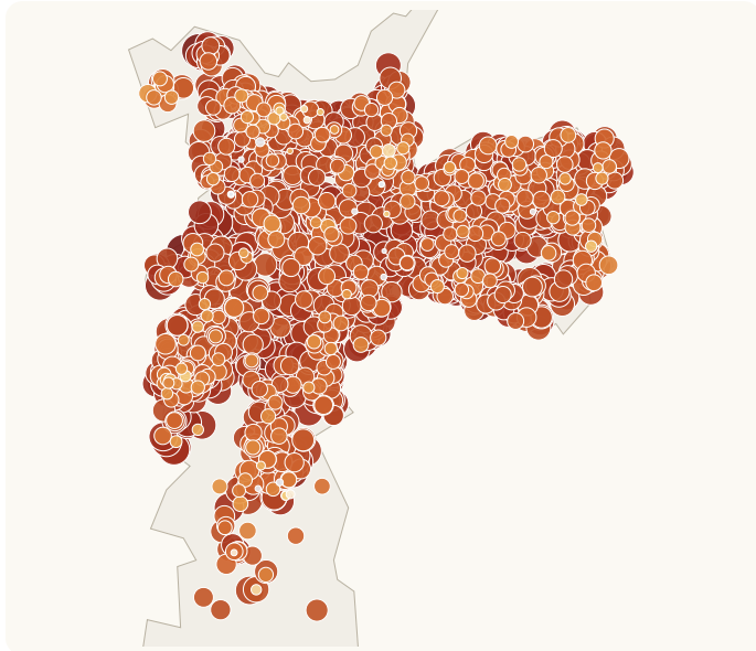
Votos por local (escala log)
